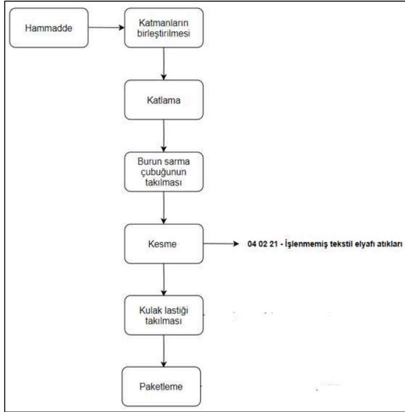
Şekil 46. Hijyenik giyim eşyası ve giysi aksesuarlarının imalatı üretim prosesi
