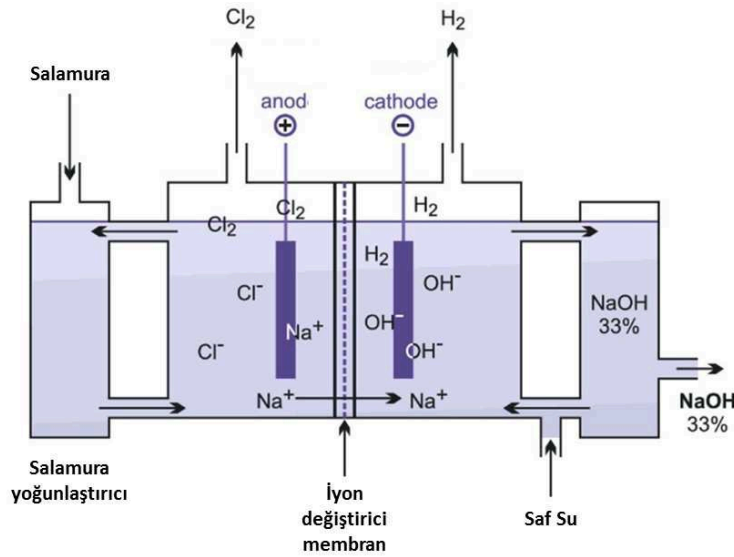
Şekil 53. Membran hücre 65
