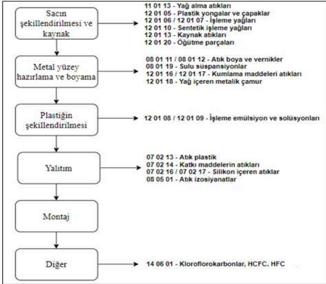
Şekil 92. Ev tipi buzdolabı, dondurucu, çamaşır makinesi, çamaşır kurutma makinesi, bulaşık makinesi, vantilatör, aspiratör, fan, aspiratörlü davlumbaz, fırın, ocak, mikrodalga fırın, elektrikli pişirme sacı vb. imalatı atık oluşum noktaları
