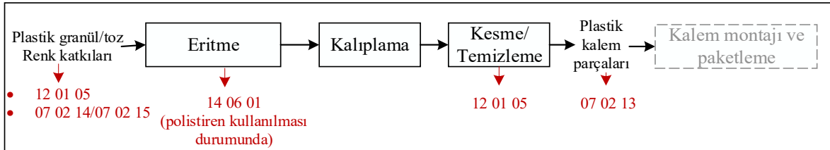
Şekil 104. Plastik kalem parçalarının imalat süreci ve atıklar
