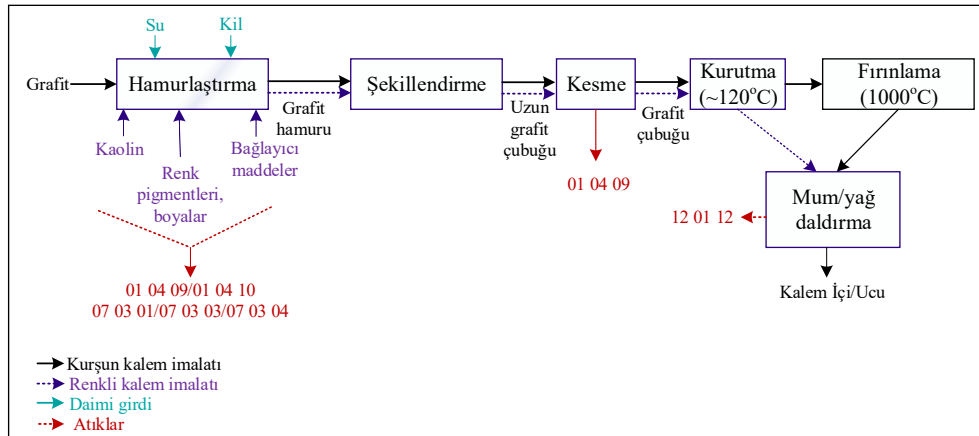
Şekil 102. Kurşun kalem ucu ve kalem içi imalat süreci ve atıklar
