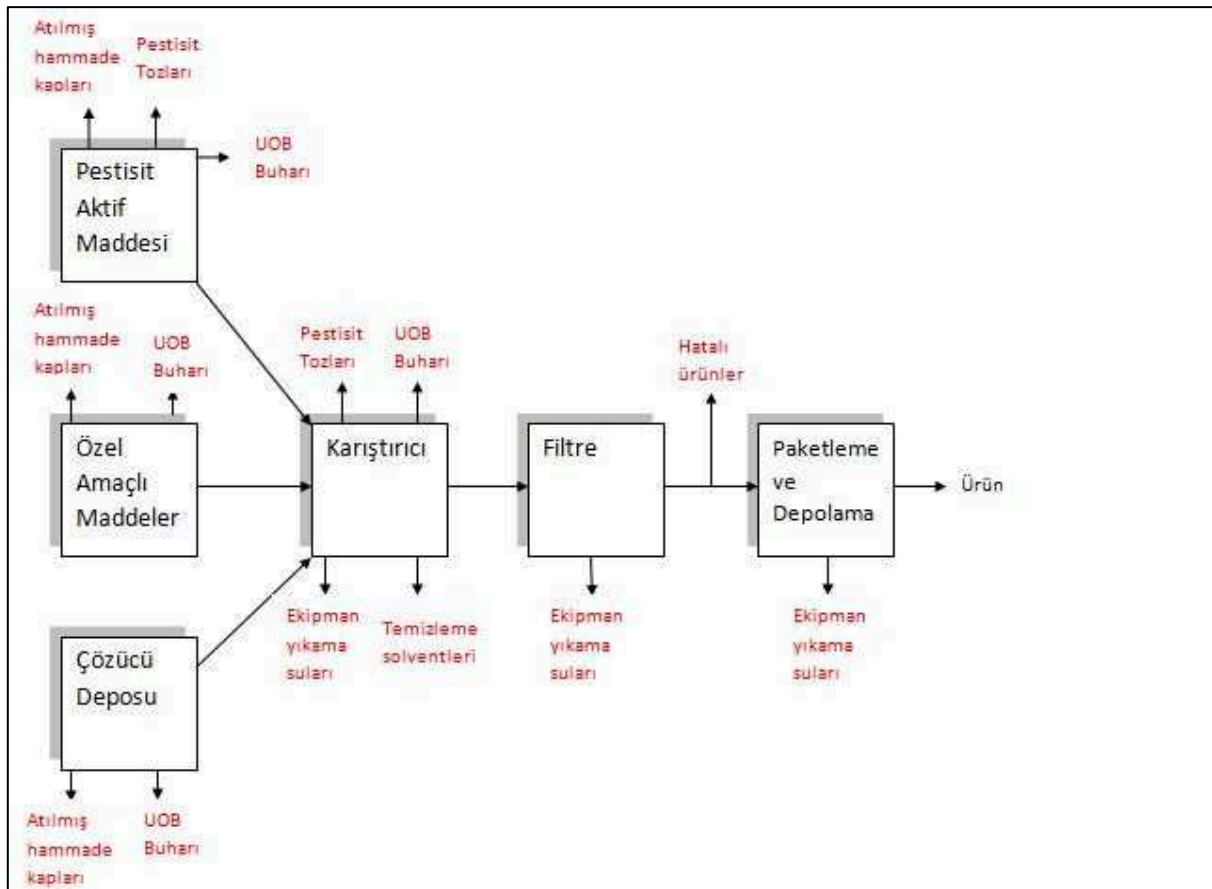
Şekil 56. Sıvı böcek ilacı, kemirgen ilacı, küf ve mantar ilacı ve yabancı otlar mücadelesine ilacı üretimi atık oluşum noktaları
