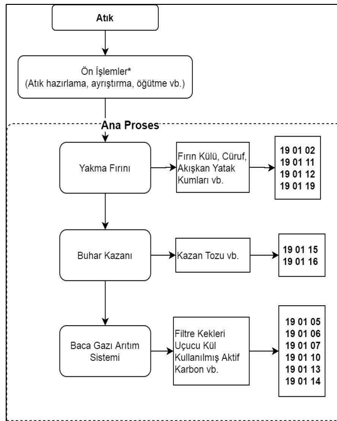
Şekil 119. Atık yakma proses 168
