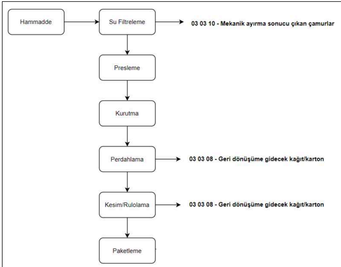
Şekil 39. Kağıt ve mukavva üretim prosesi
