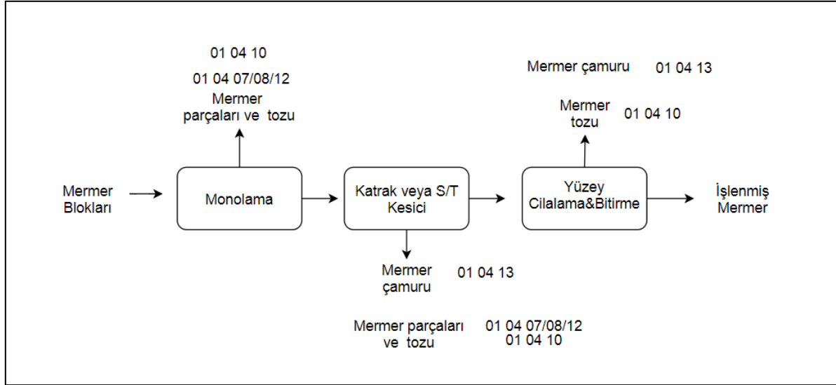
Şekil 76. Tas ve mermer üretim prosesi
