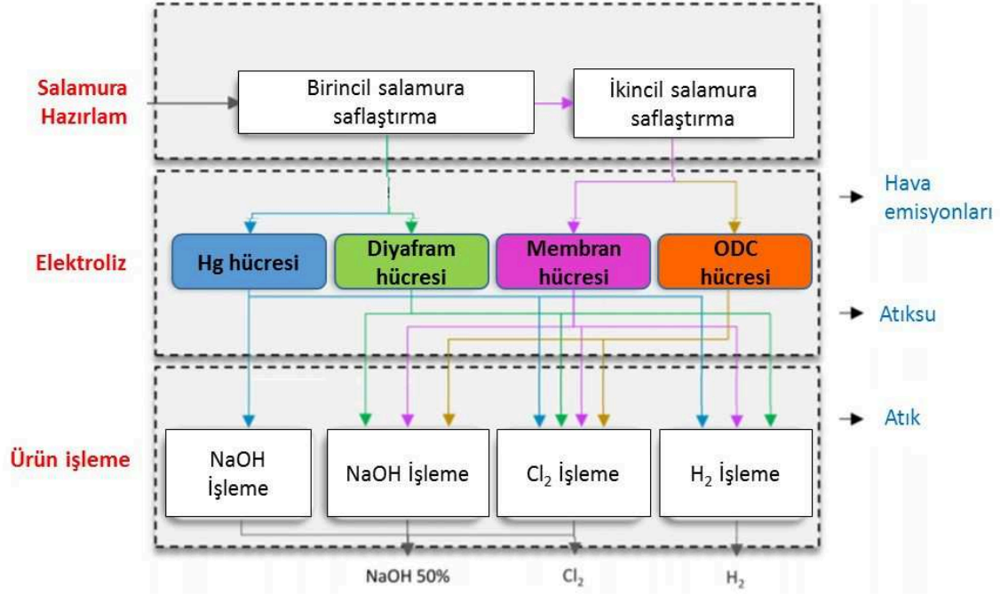
Şekil 49. Klor-alkali prosesleri 61
