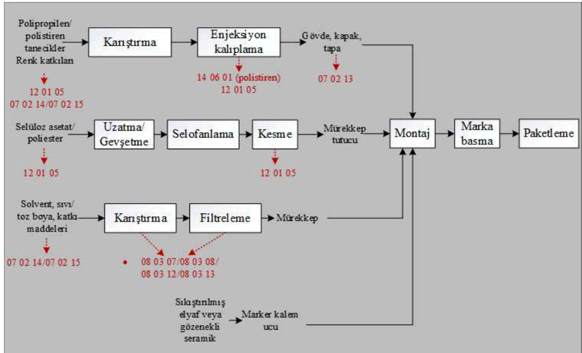
Şekil 112. Marker kalem imalat süreci ve atık noktaları
