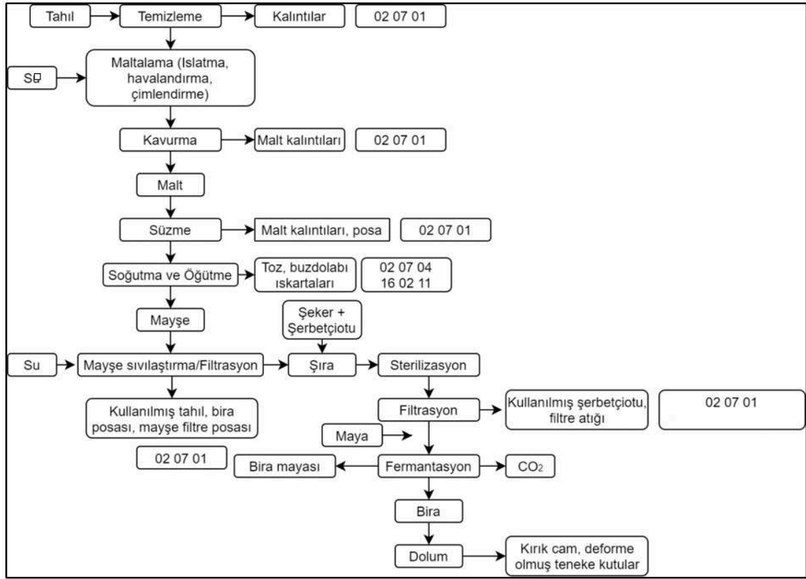
Şekil 6. Bira üretimi akım şeması ve kaynaklanan proses atıkları 24
