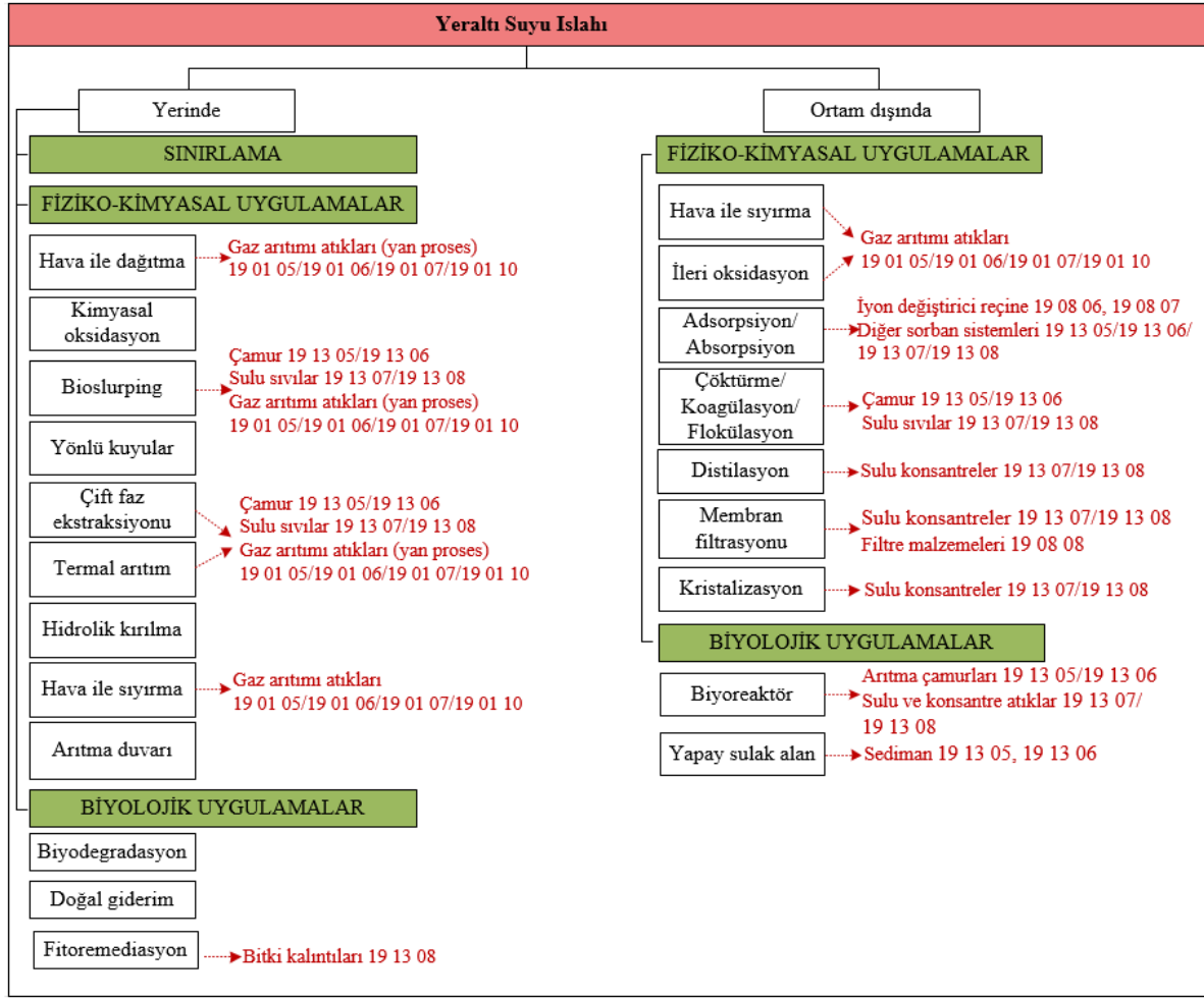
Şekil 137. Yeraltı suyu ıslahı prosesleri ve atıklar
