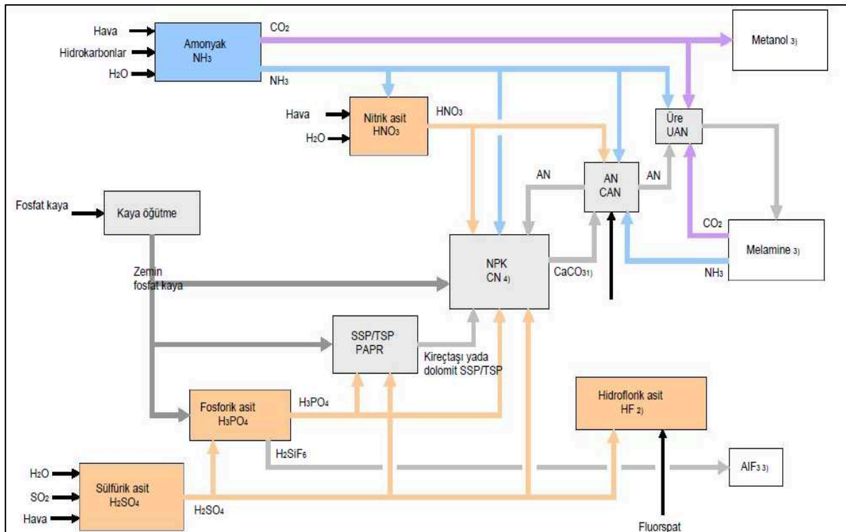
Şekil 54. Amonyak, gübre ve asit endüstrileri arasındaki sınırlar ve bağlantılar hakkında genel bilgi
