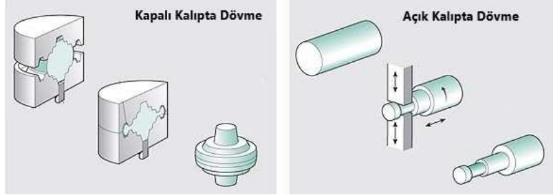
Şekil 86. Açık ve kapalı kalıp dövme işlemi 100
