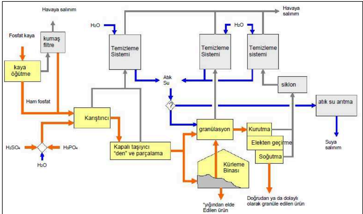
Şekil 55. Süper fosfat üretimi hakkında genel prosesler (atık gaz arıtma sistemi dahil)
