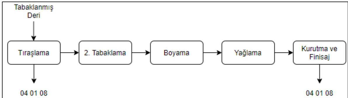
Şekil 34. Tabaklanmış deri işleme sektörü atık oluşum noktaları
