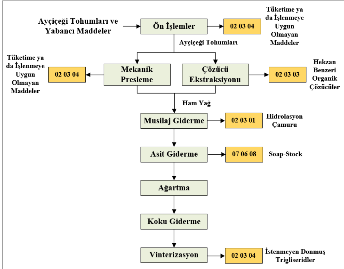
Şekil 1. Ayçiçek yağı üretim prosesi 3
