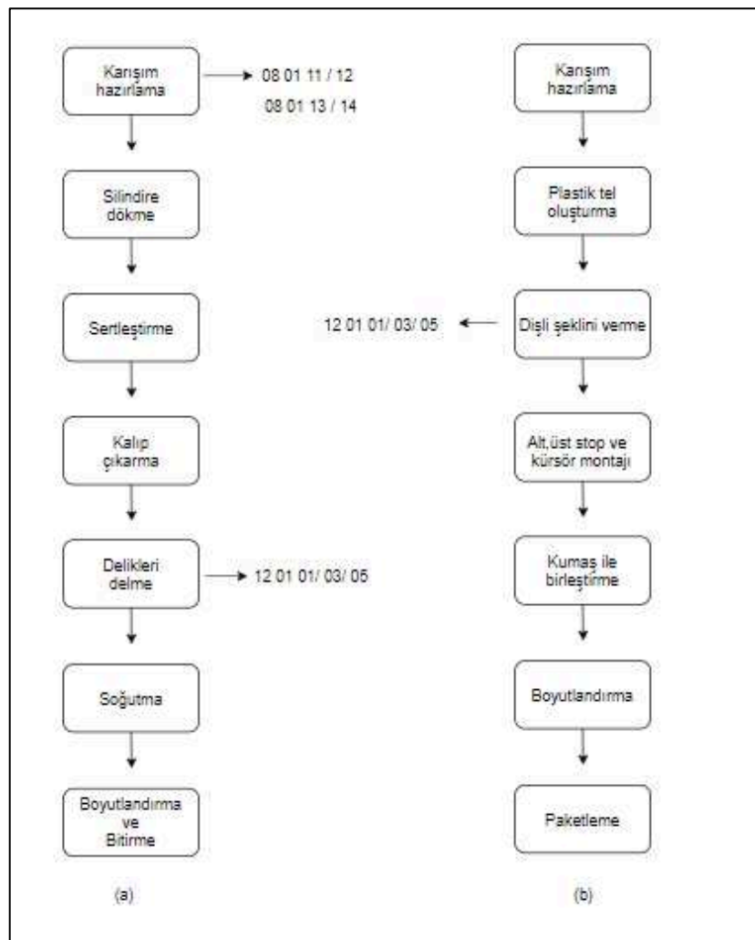
Şekil 101. Kot vb. baskı düğmeleri, çıtçıtlar, düğmeler, fermuarlar vb. imalatı üretim prosesi
