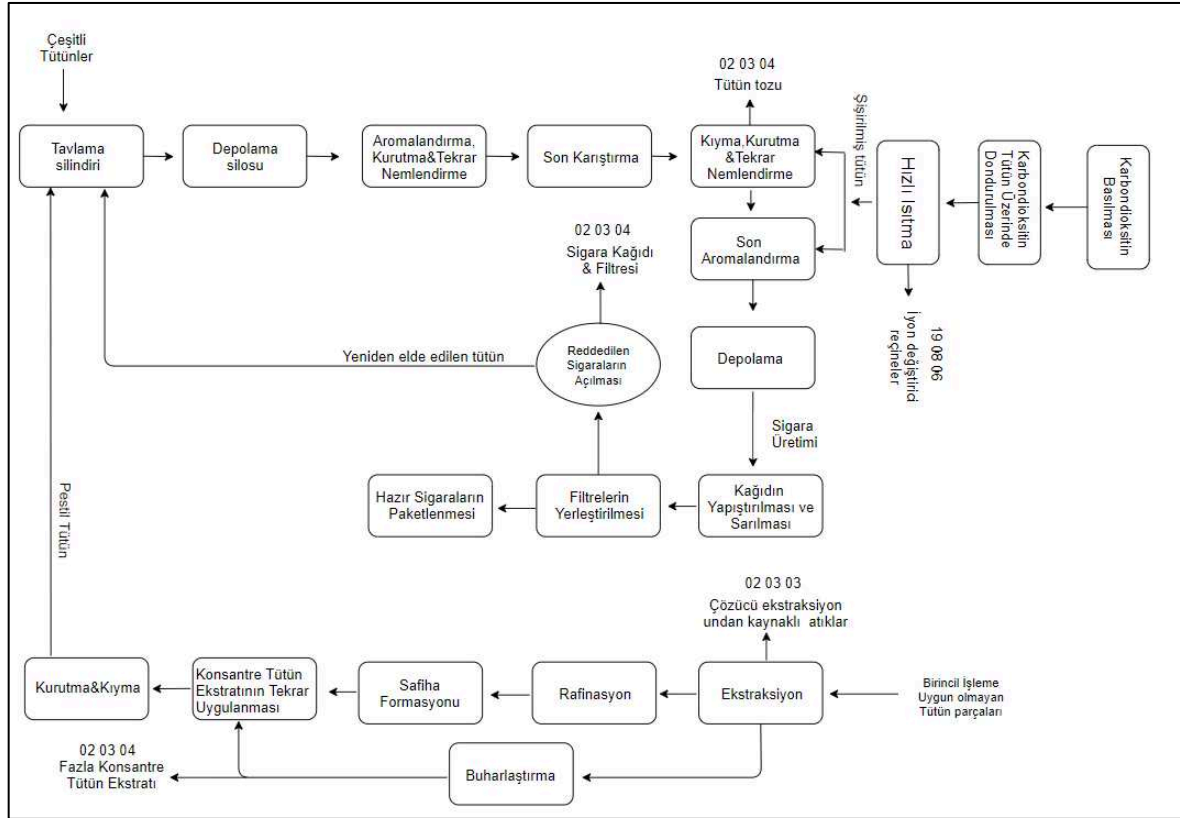
Şekil 9. Sigara üretim prosesi
