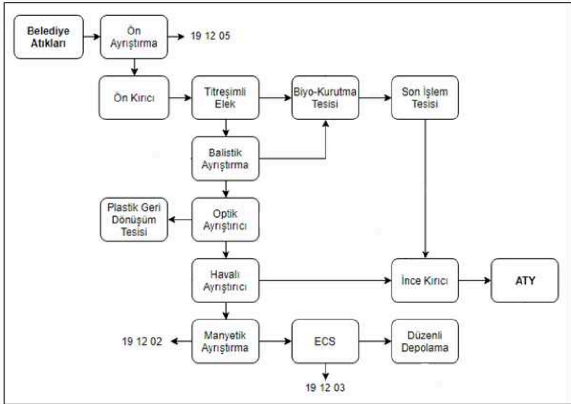
Şekil 126. ATY hazırlama akım şeması
