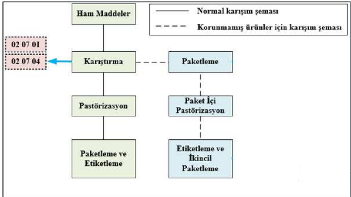
Şekil 8. Gazsız alkolsüz içecek üretimi akım şeması ve kaynaklanan proses atıkları
