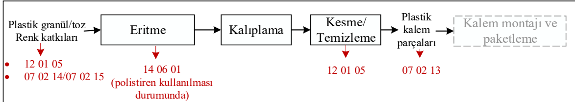
Şekil 107. Plastik kalem parçalarının imalat prosesi ve atıklar
