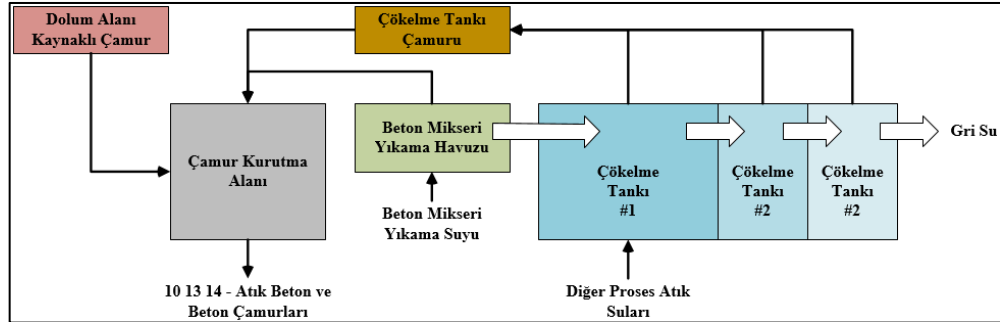
Şekil 75. Hazır beton tesisi atıksu arıtma prosesi akım şeması 88
