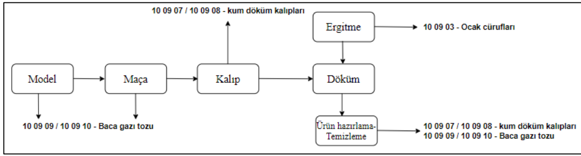
Şekil 83. Demir döküm tesislerinde atık oluşum noktaları
