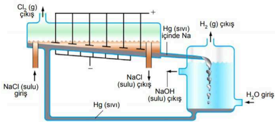
Şekil 51. Cıva hücresi 63
